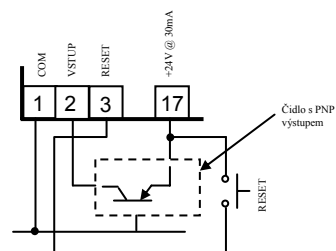
Příklad připojení čidla s výstupem PNP
