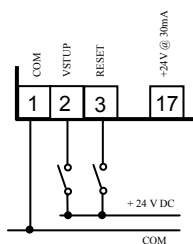
napěťový vstup
